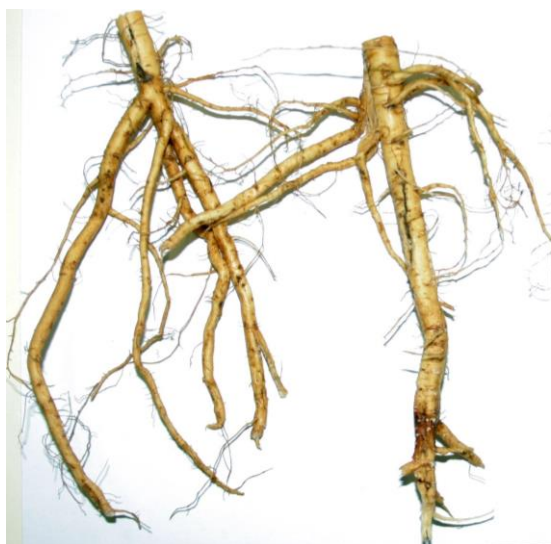
Obrázek 3 Příklady intenzivního větvení kořenového systému vojtěšky seté.
